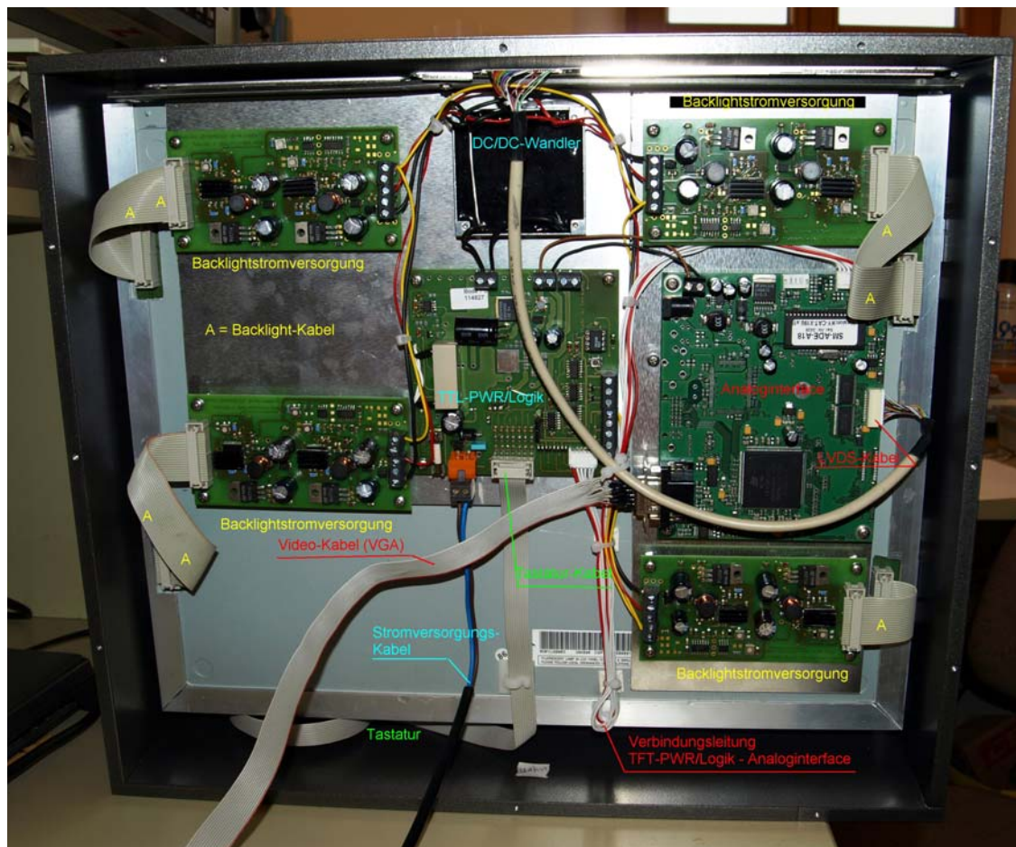
Abb. 3 Anordnung der Elektronik-Baugruppen
