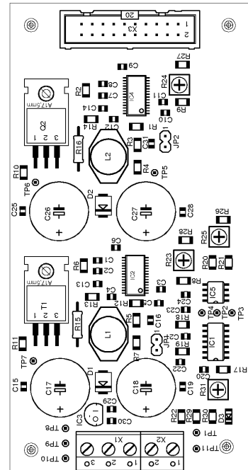
Abb. 7 Bestückungsplan LED-Backlightstromversorgung
